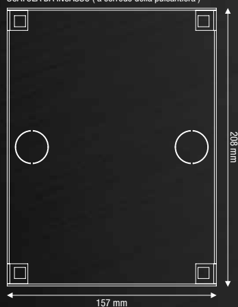
SCATOLA DA INCASSO ( a corredo della pulsantiera )
