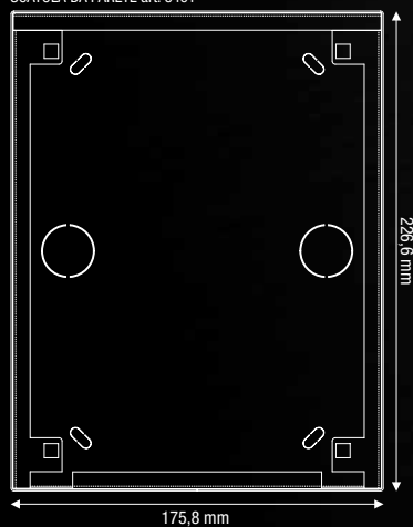
SCATOLA DA PARETE art. 3461
