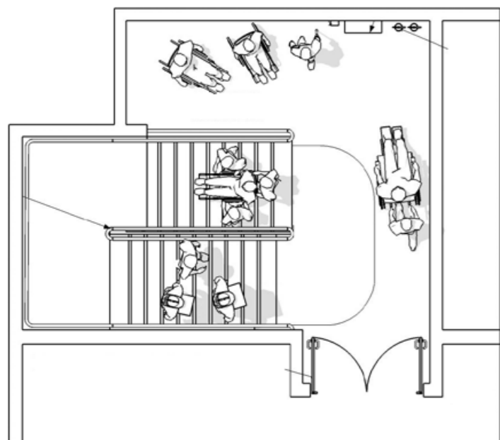
ESEMPIO DI SPAZIO CALMO: (AREA OF RESCUE ASSISTANCE) SECONDO NORMA ISO 21542
